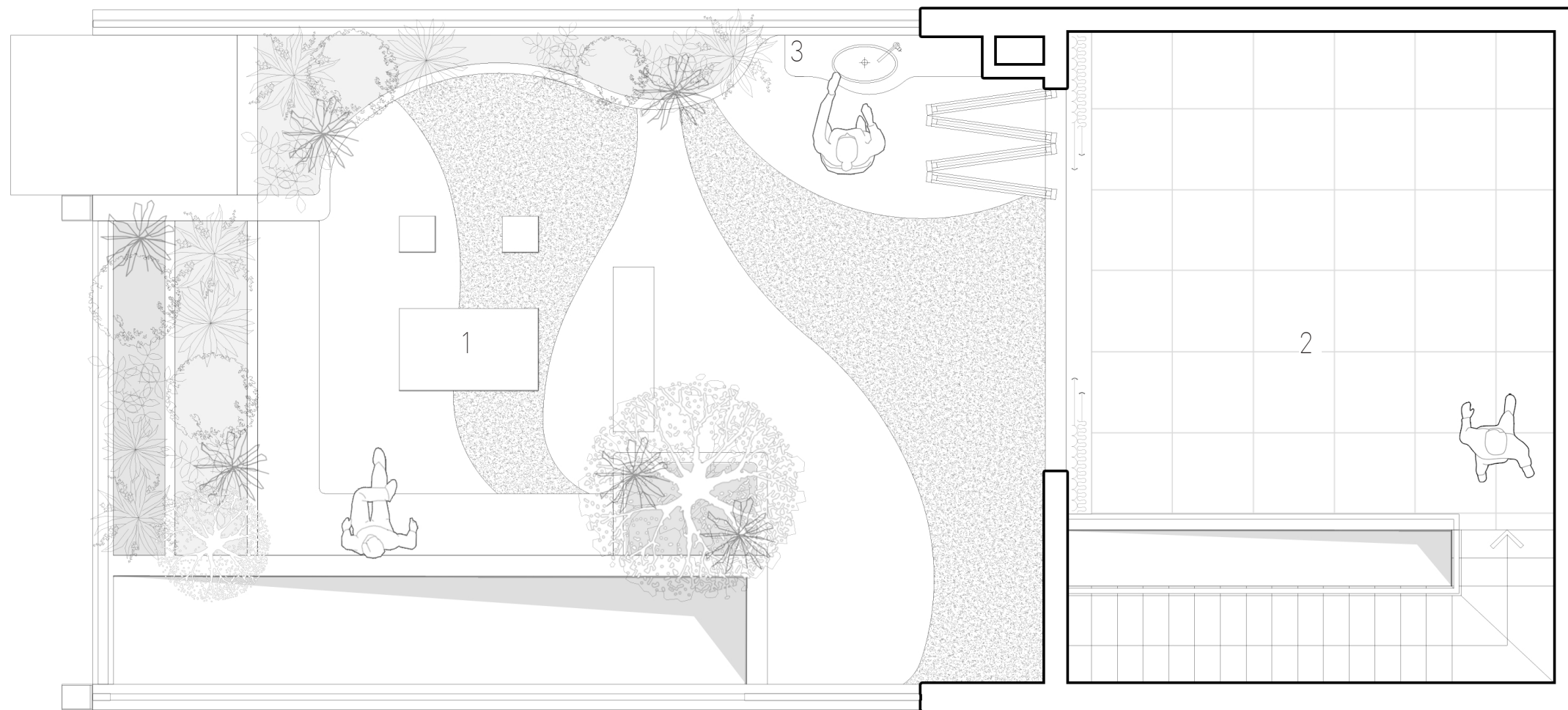
MẶT BẰNG TẦNG THƯỢNG | TERRACE FLOOR PLAN
