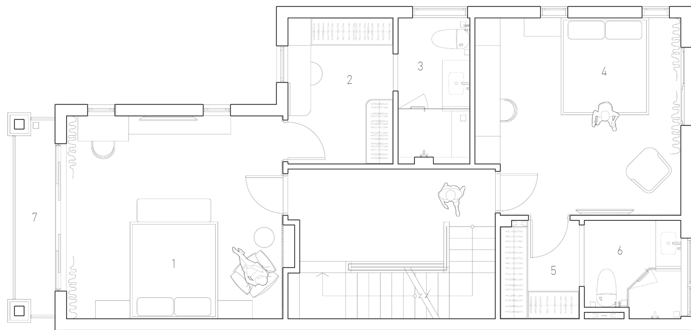
MẶT BẰNG TẦNG HAI | 2ND FLOOR PLAN
