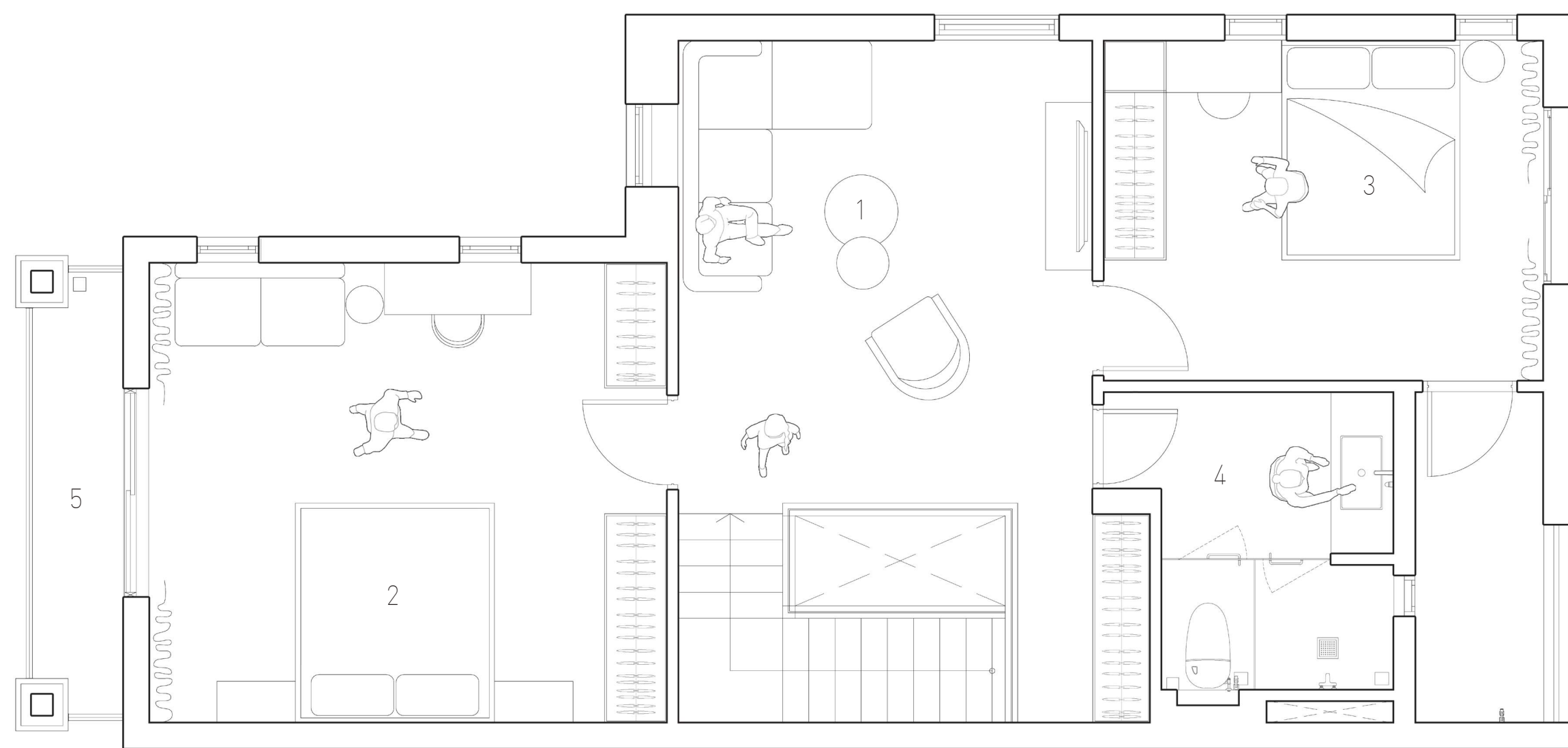
MẶT BẰNG TẦNG BA | 3RD FLOOR PLAN
