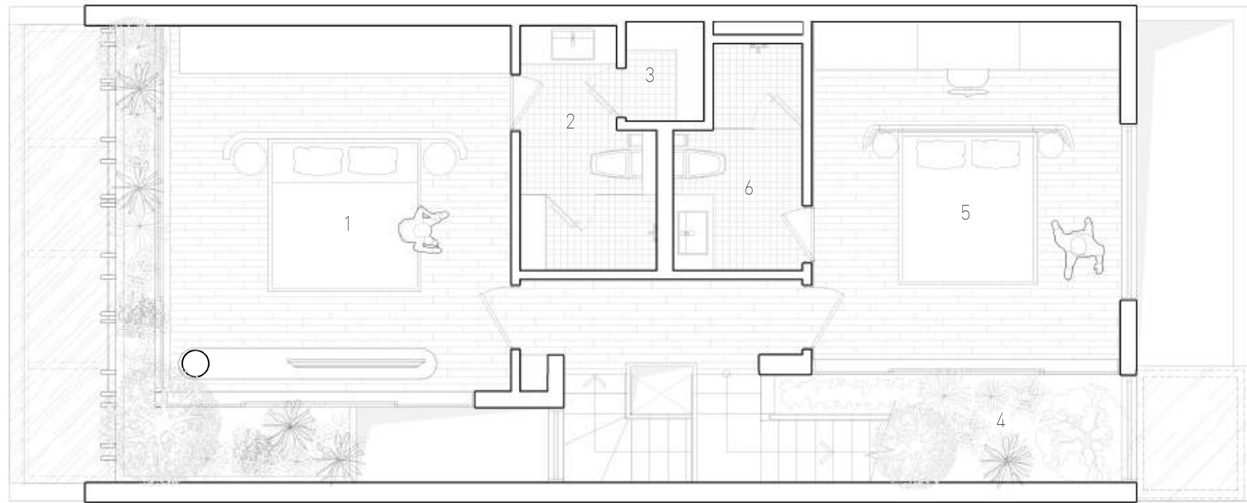
MẶT BẰNG TẦNG HAI | 2ND FLOOR PLAN
