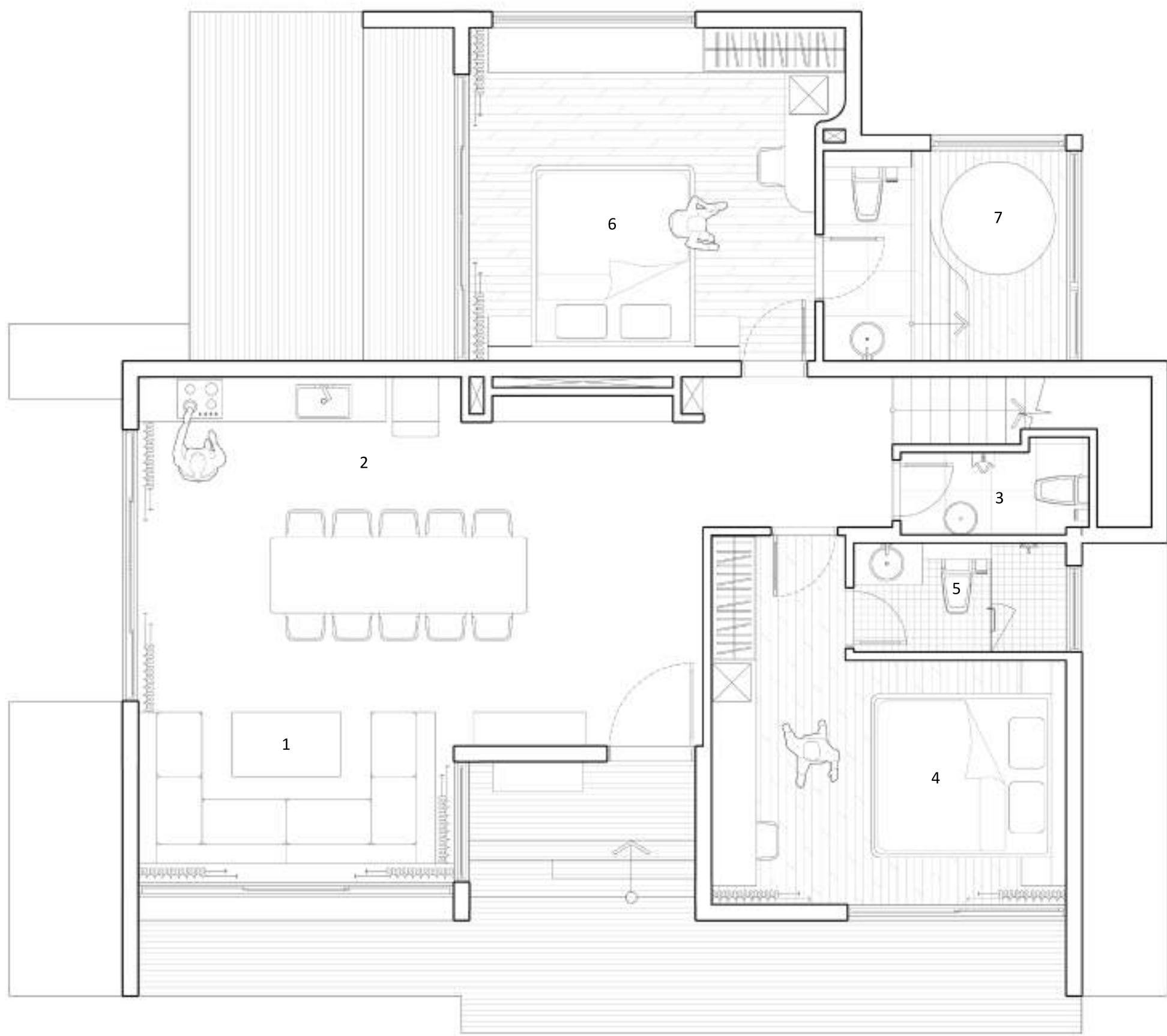
MẶT BẰNG TẦNG TRỆT | GROUND FLOOR PLAN
