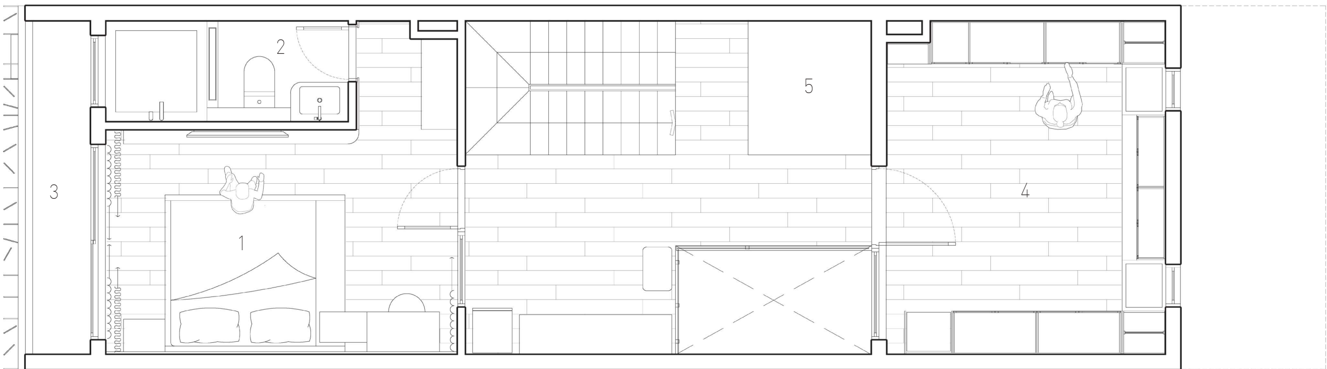
MẶT BẰNG TẦNG BA | 3RD FLOOR PLAN
