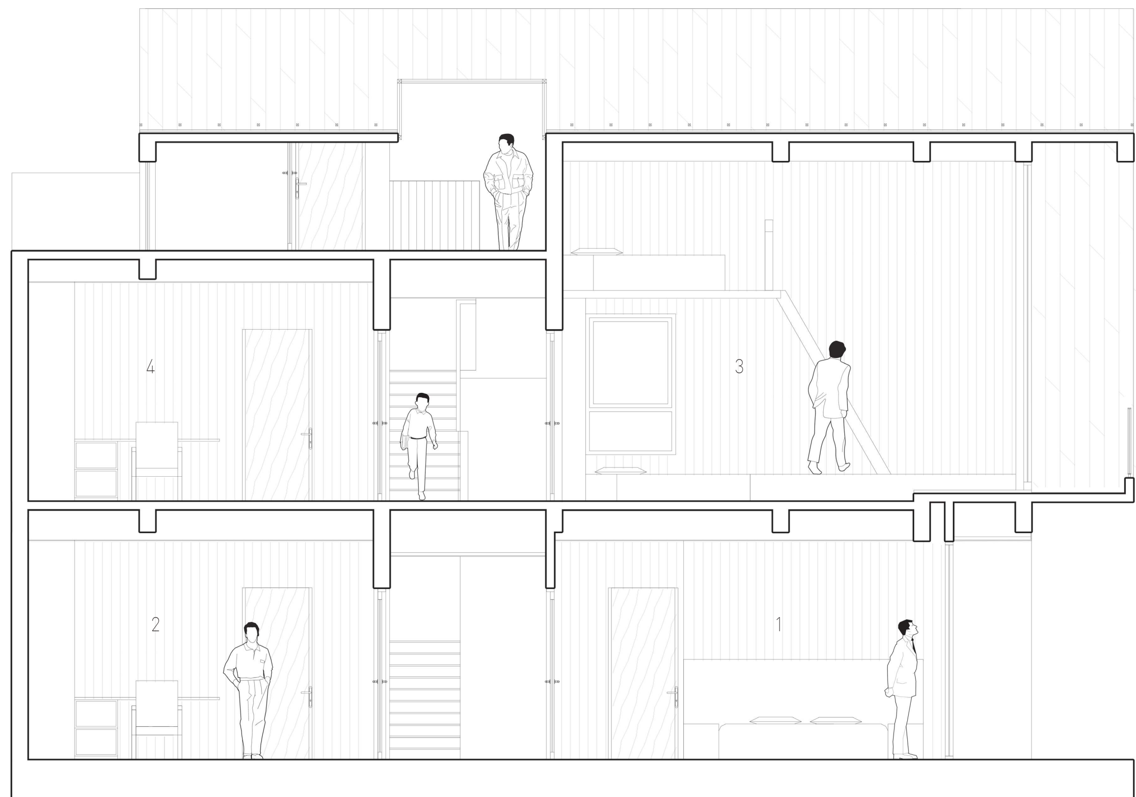
MẶT CẮT 2 | SECTION 2
