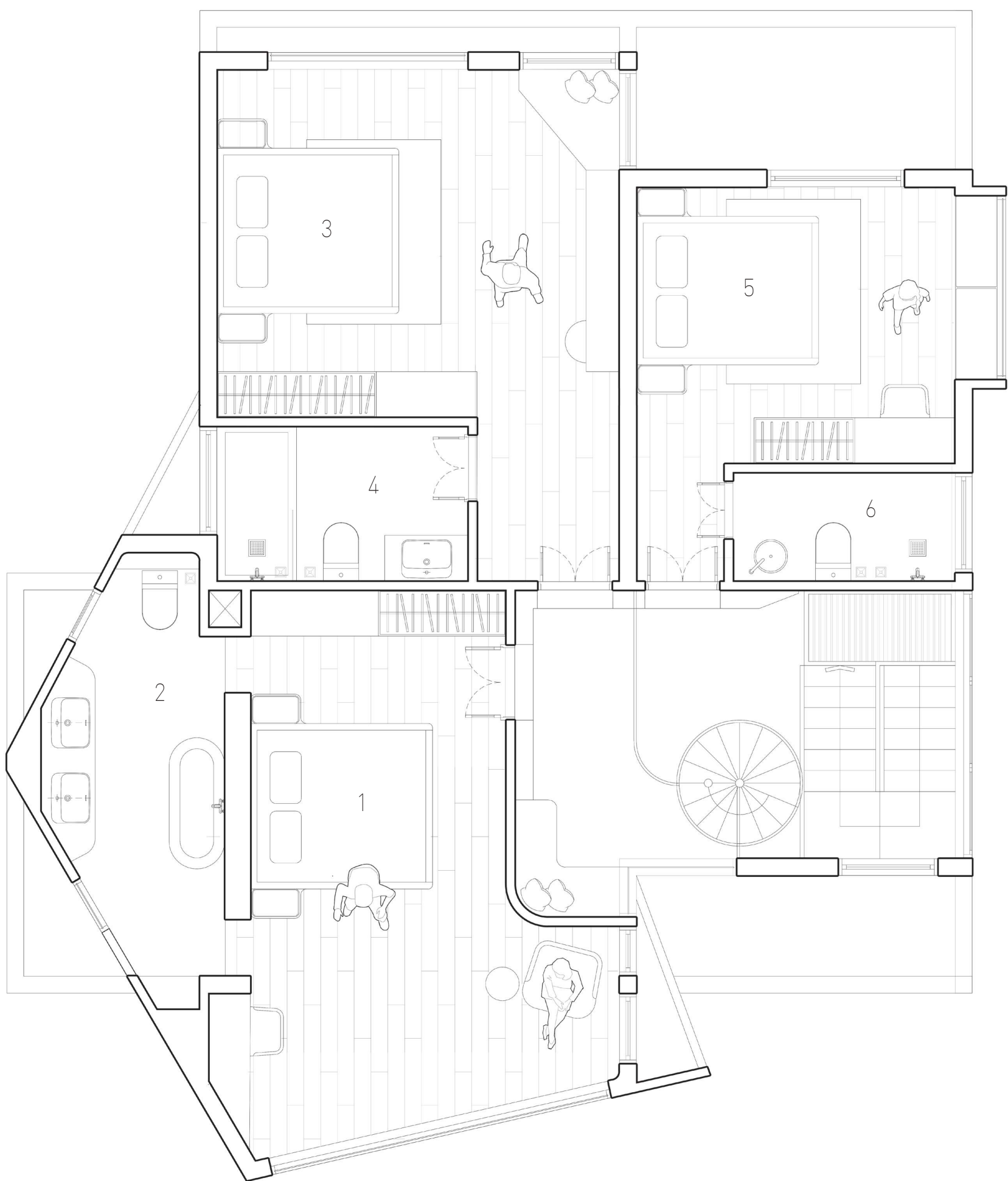
MẶT BẰNG TẦNG HAI | 2ND FLOOR PLAN
