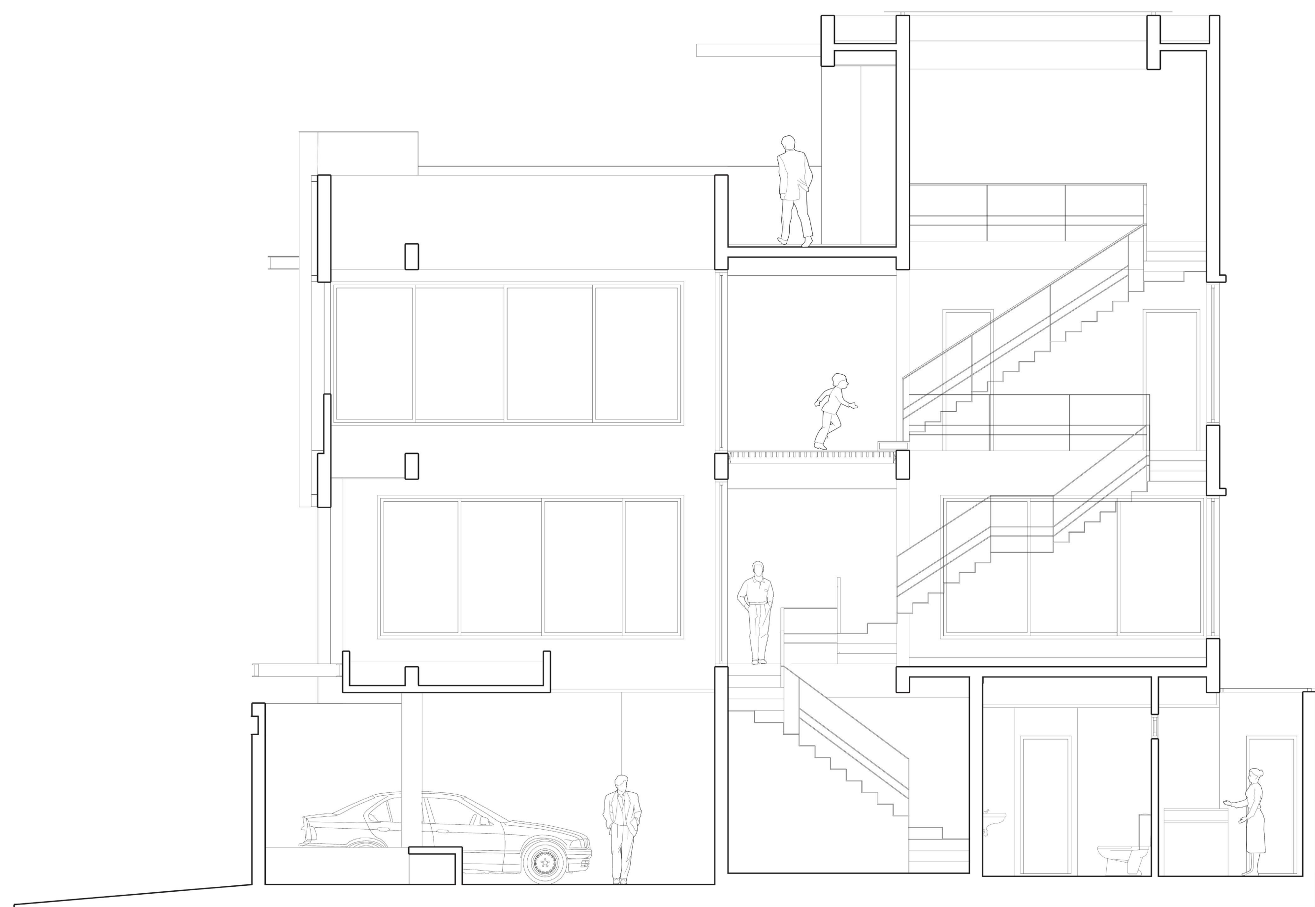
MẶT CẮT 1 | SECTION 1
