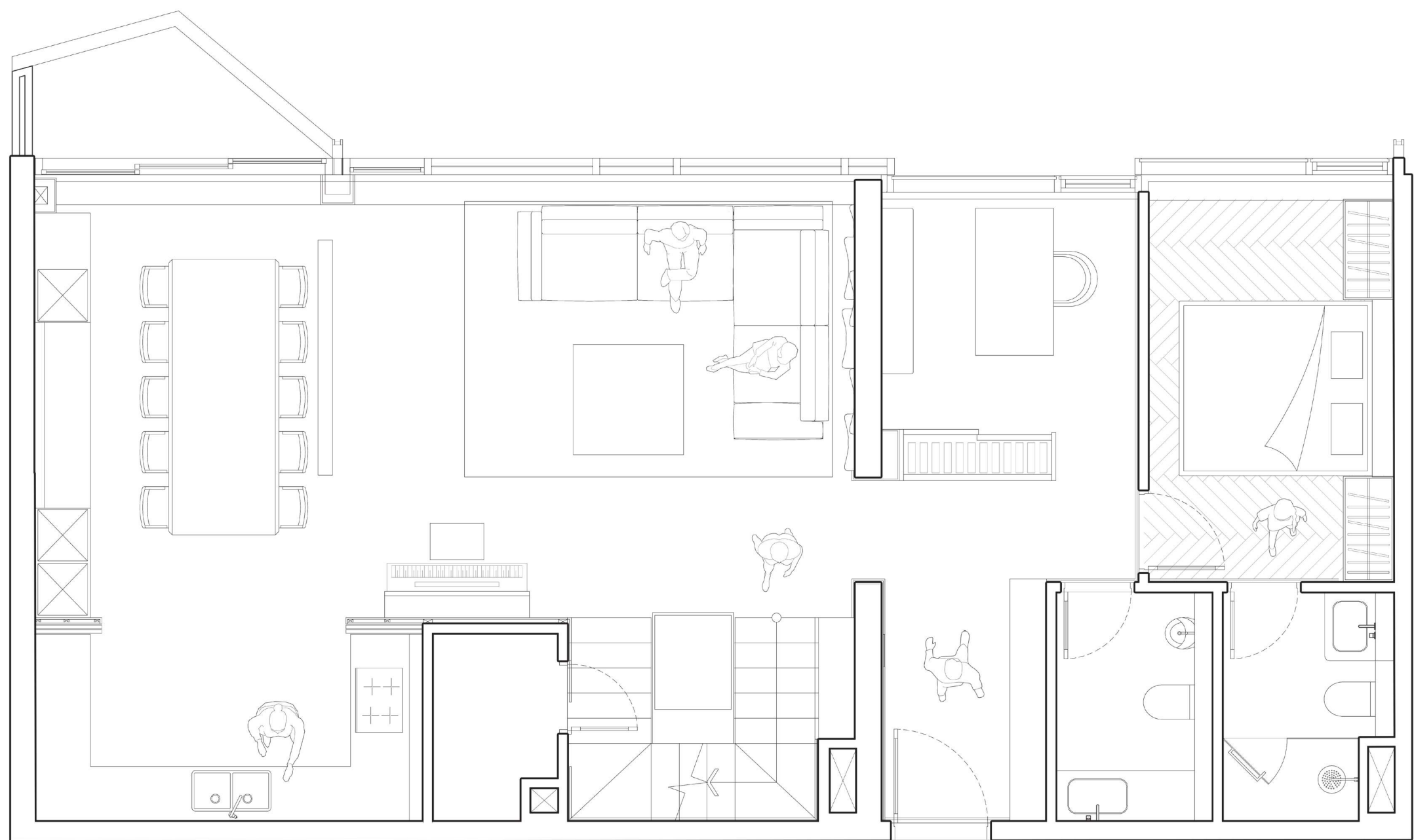
MẶT BẰNG TẦNG TRỆT | GROUND FLOOR PLAN
