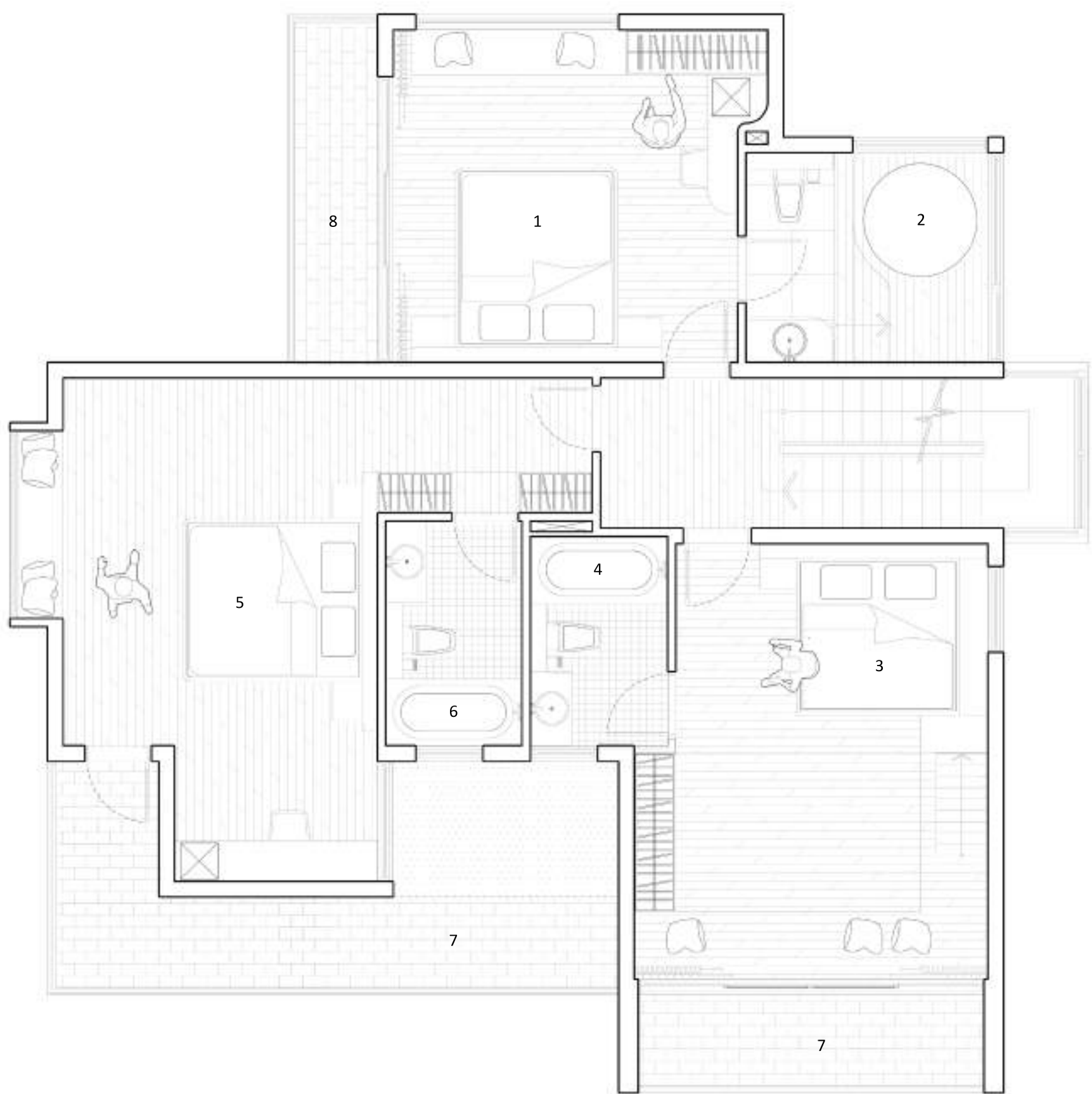
MẶT BẰNG TẦNG HAI | 2ND FLOOR PLAN
