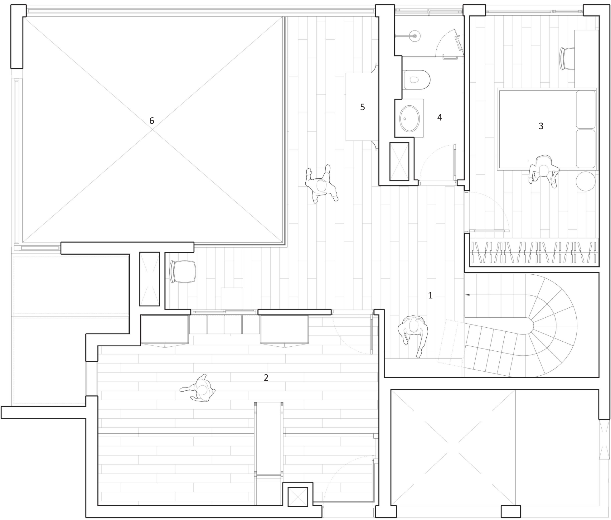
MẶT BẰNG TẦNG 22 | 22ST FLOOR PLAN
