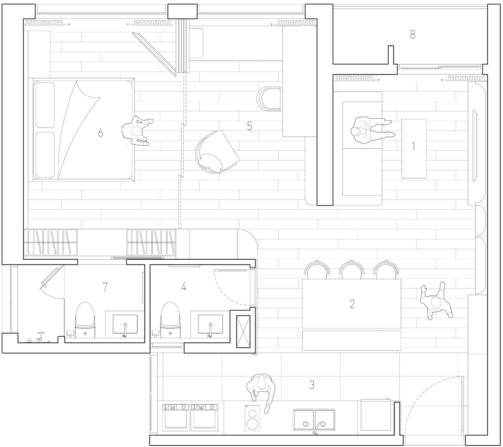
MẶT BẰNG BỐ TRÍ VẬT DỤNG | FLOOR PLAN
