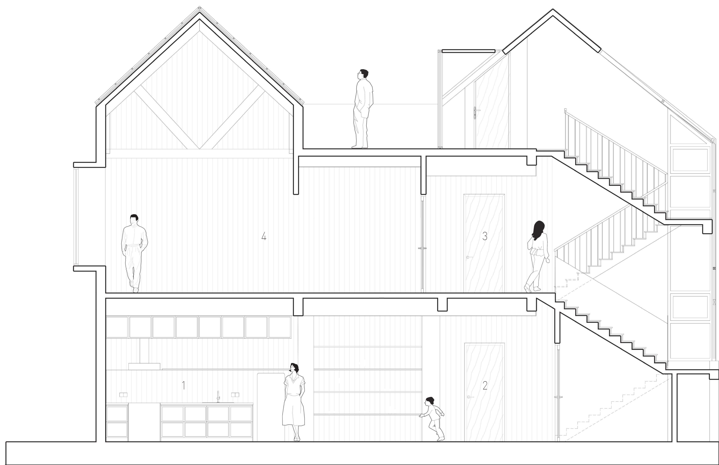
MẶT CẮT 1 | SECTION 1
