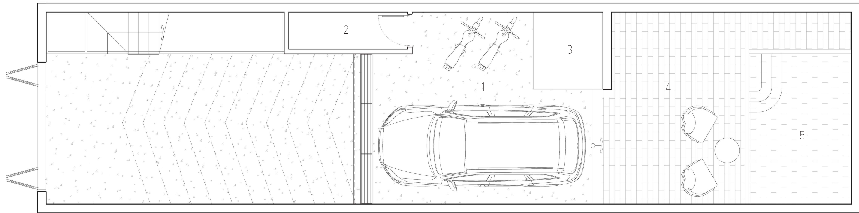
MẶT BẰNG TẦNG HẦM | BASEMENT FLOOR PLAN
