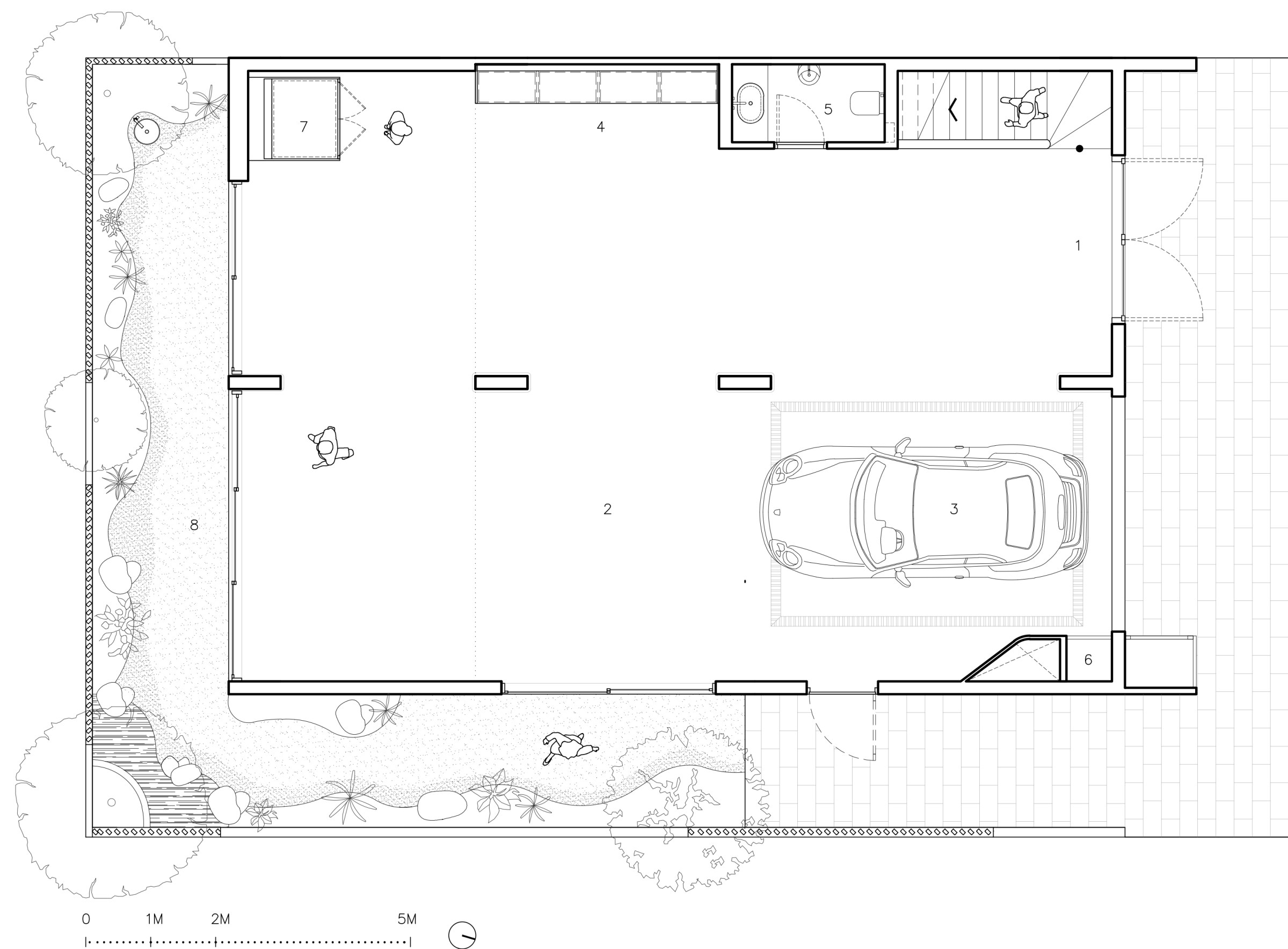
MẶT BẰNG TẦNG TRỆT | GROUND FLOOR PLAN
