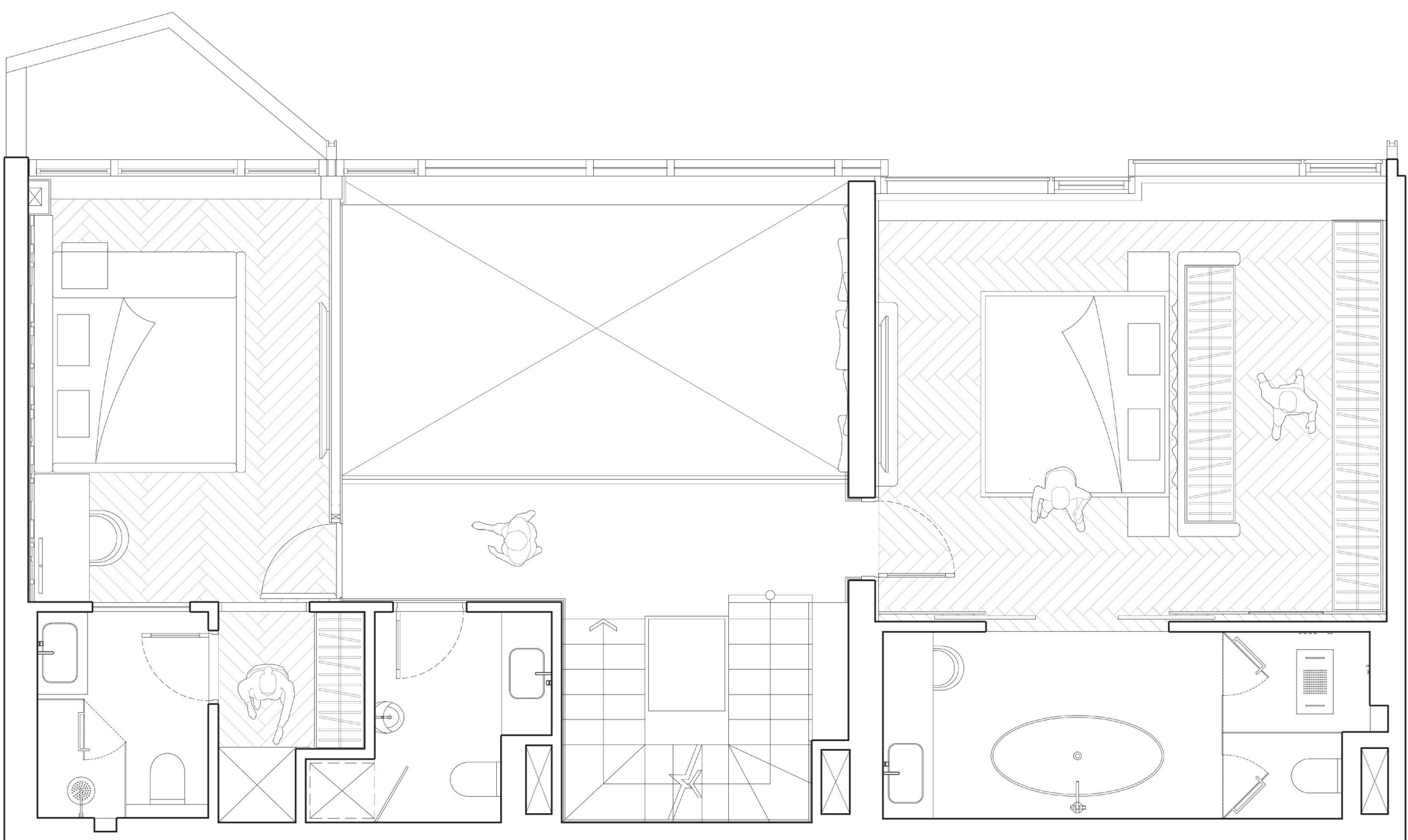
MẶT BẰNG TẦNG HAI | 2ND FLOOR PLAN
