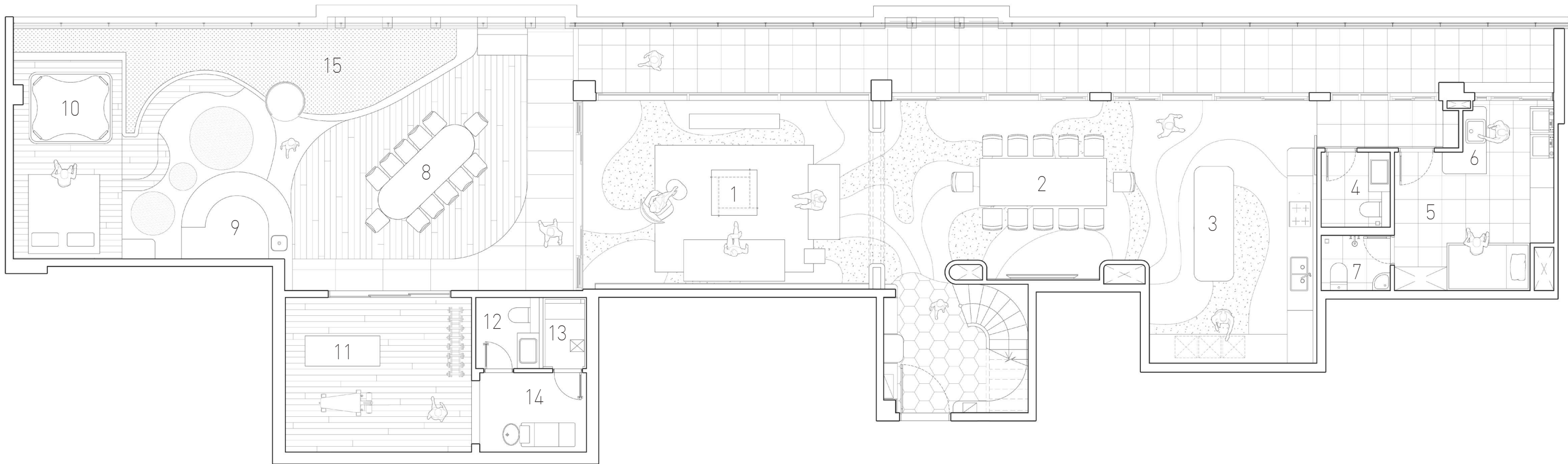
MẶT BẰNG TẦNG 40 | 40TH FLOOR PLAN
