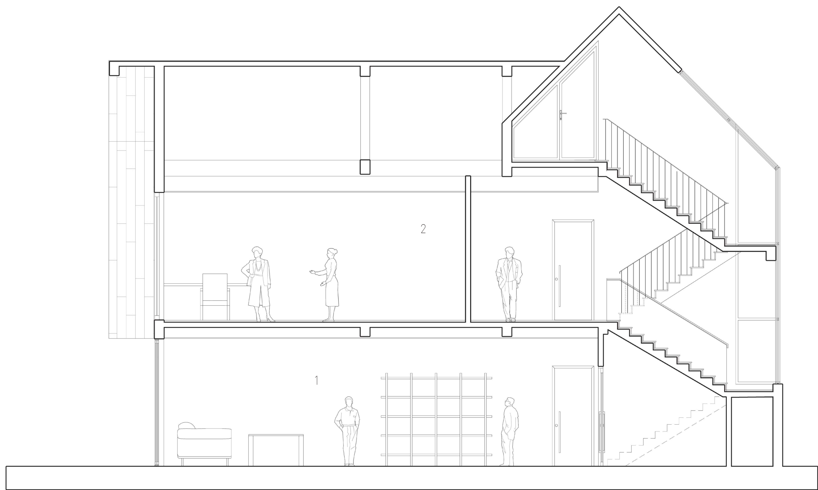
MẶT CẮT 1 | SECTION 1
