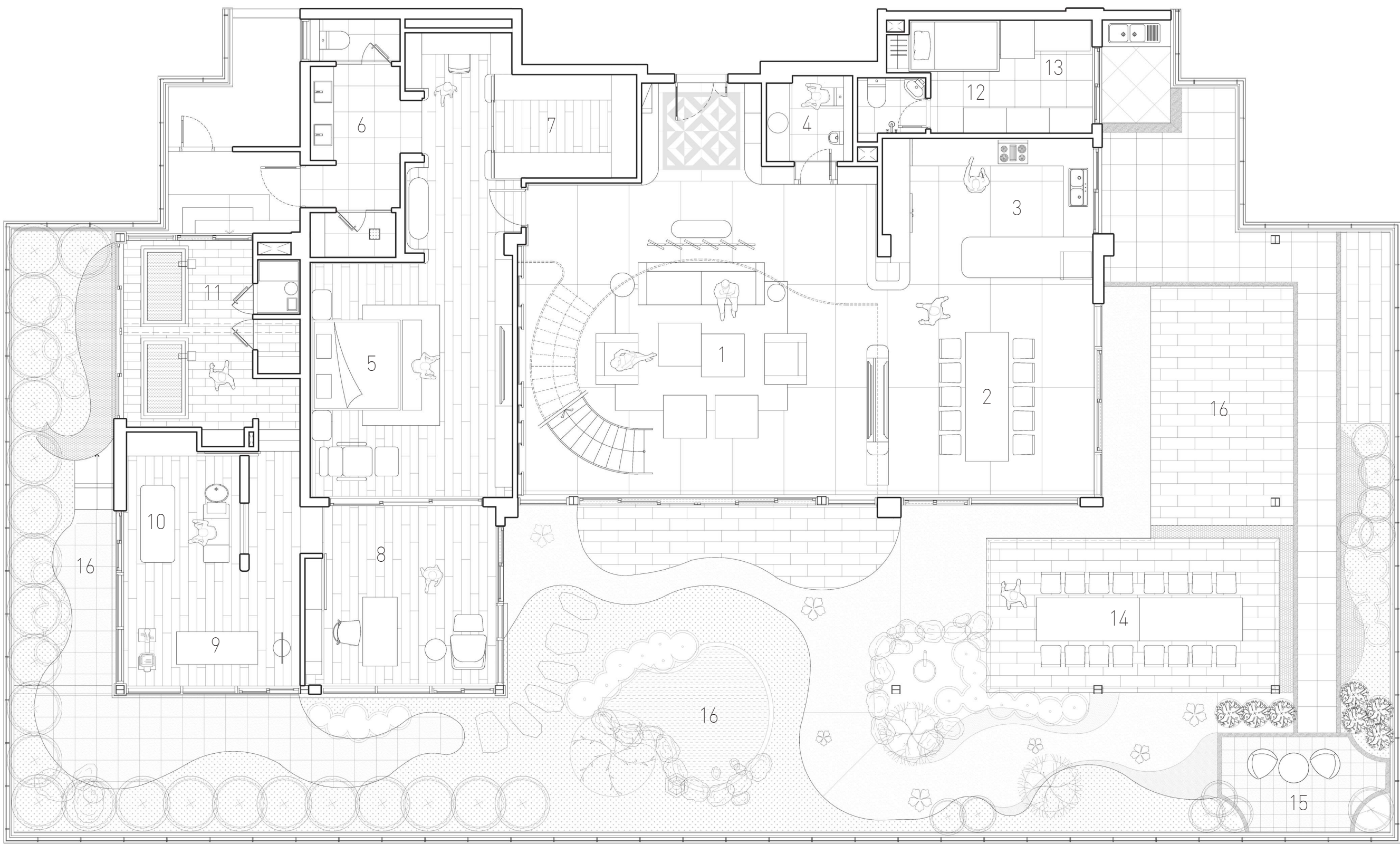
MẶT BẰNG TẦNG 40 | 40TH FLOOR PLAN
