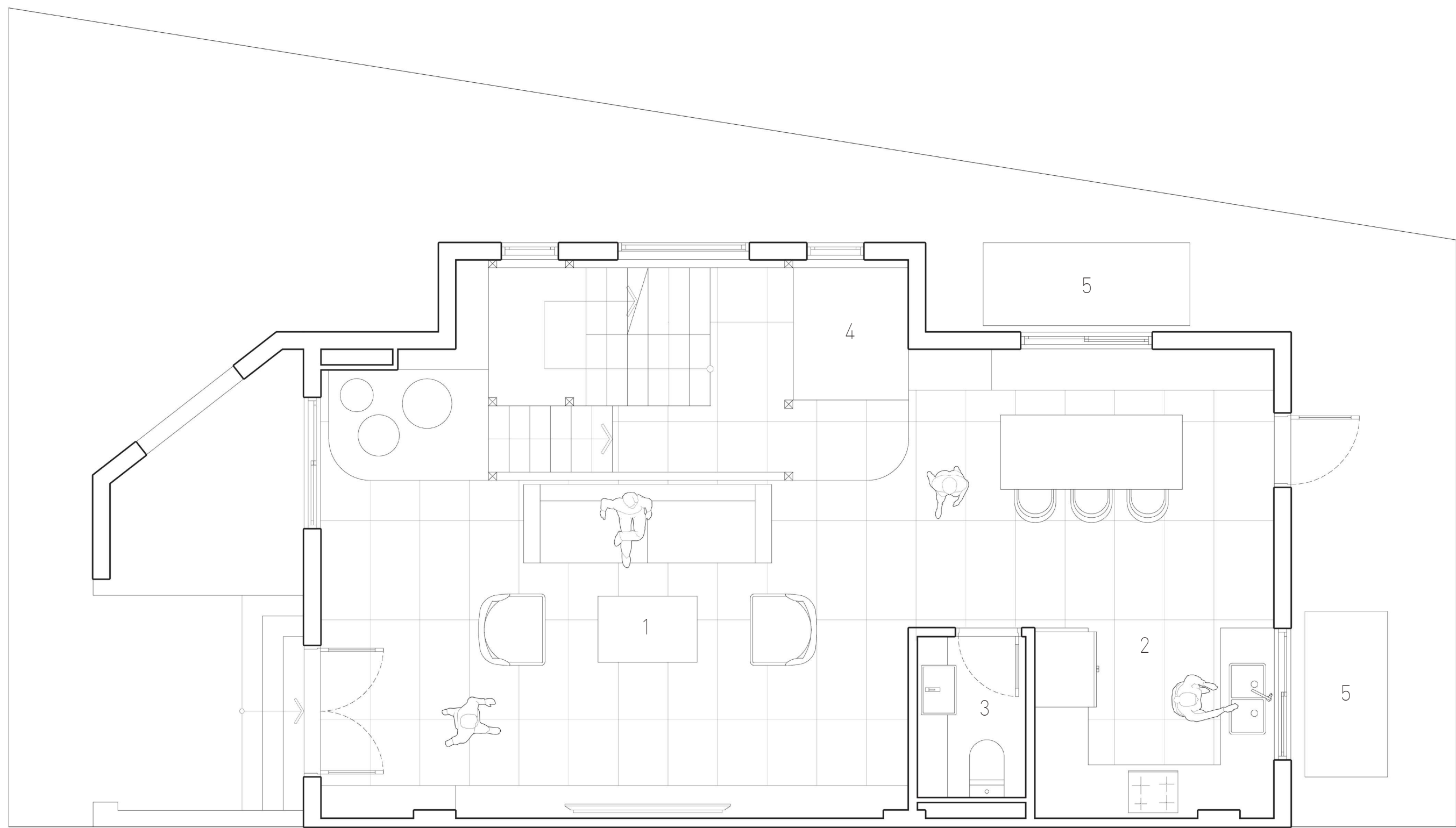
MẶT BẰNG TẦNG TRỆT | GROUND FLOOR PLAN
