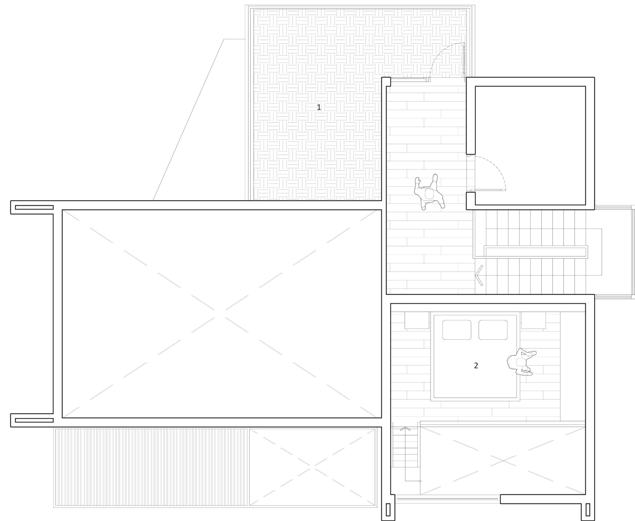
MẶT BẰNG TẦNG BA | 3RD FLOOR PLAN
