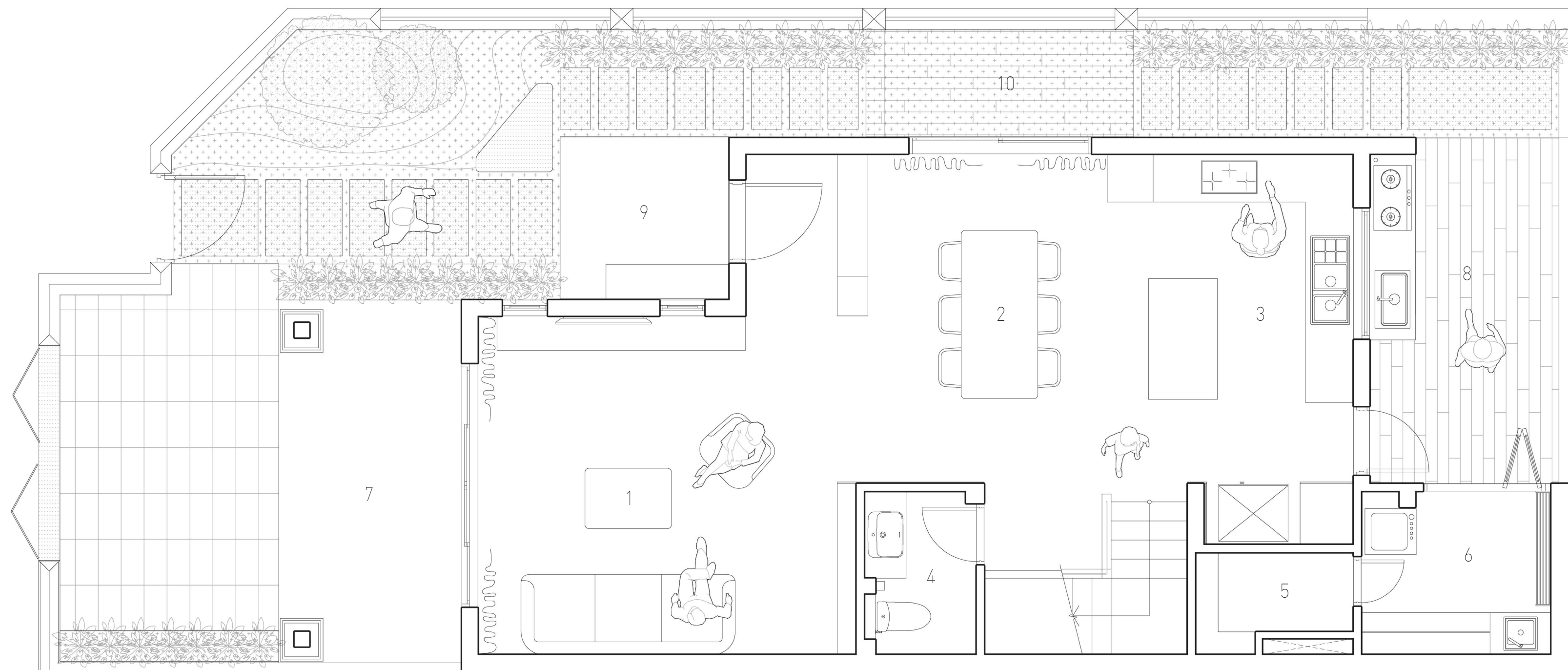
MẶT BẰNG TRỆT TỔNG THỂ | PLAN
