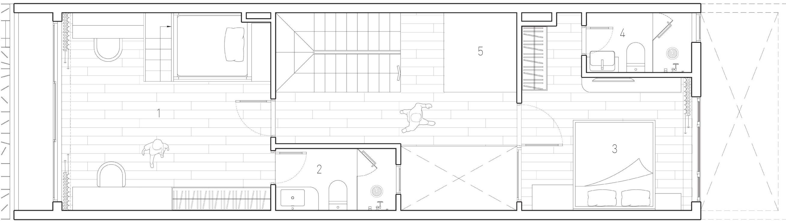
MẶT BẰNG TẦNG HAI | 2ND FLOOR PLAN
