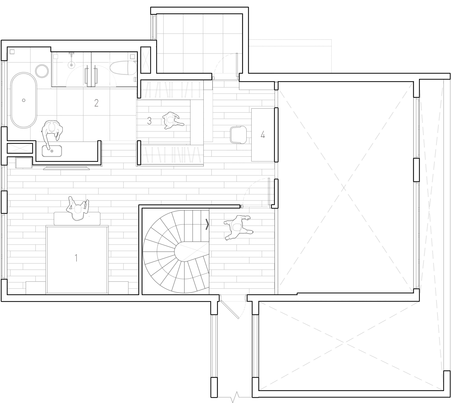
MẶT BẰNG TẦNG HAI | 2ND FLOOR PLAN
